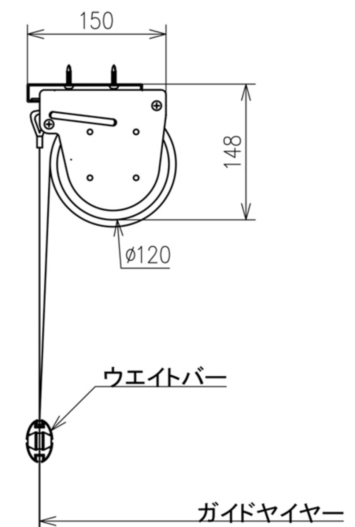
側面図
