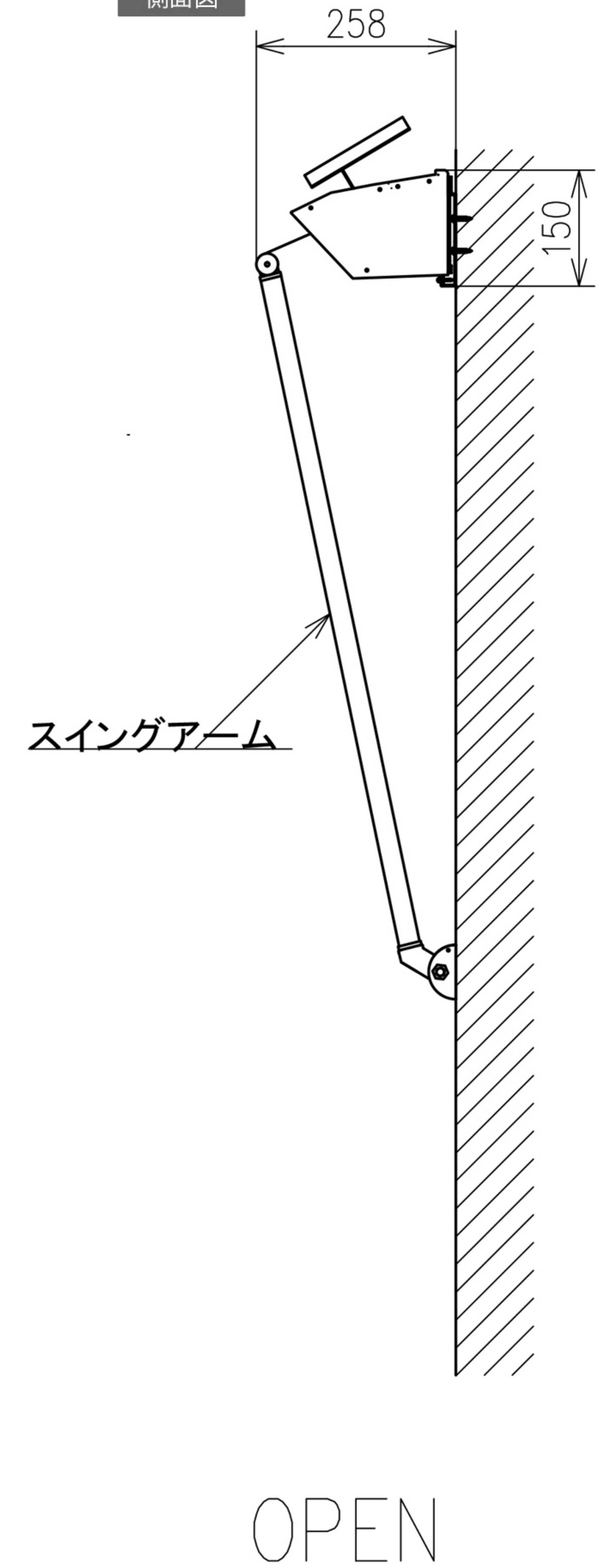
側面図
