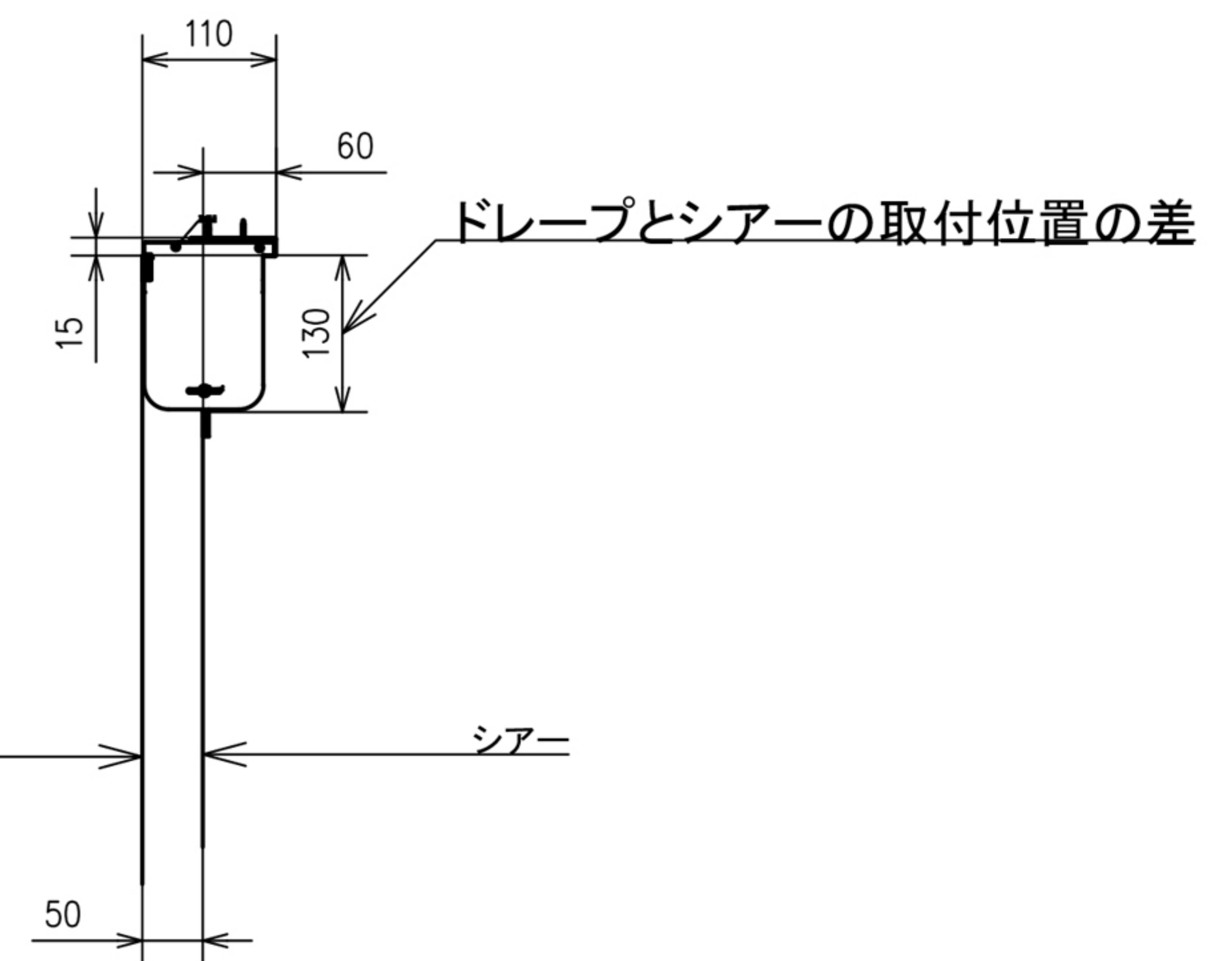
側面図
