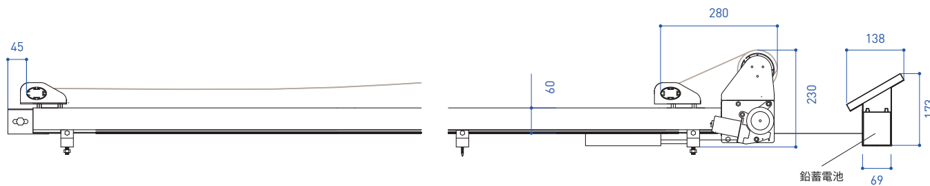
正面図
