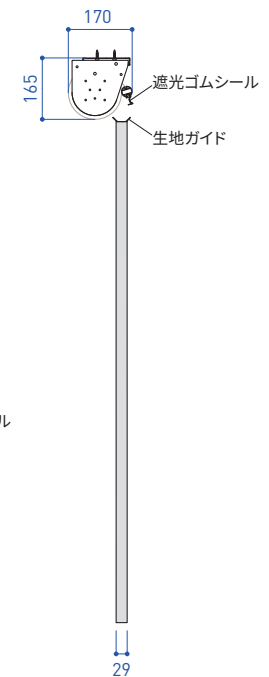
側面図
