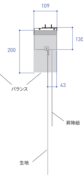
側面図
