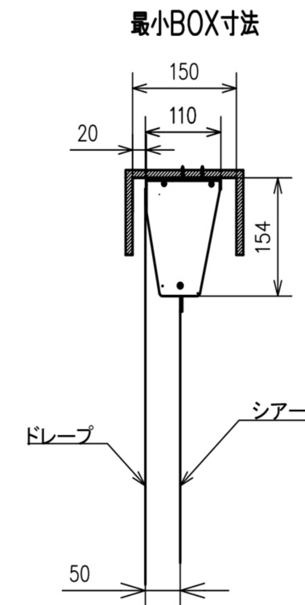
側面図
