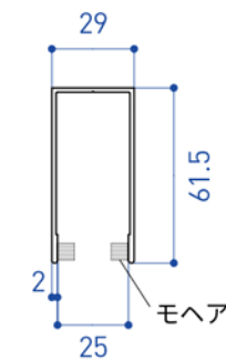
遮光ガイドレール 断面図
